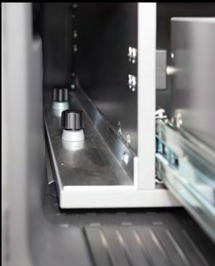
Detail der Verriegelungspunkte der Heckschublade.
