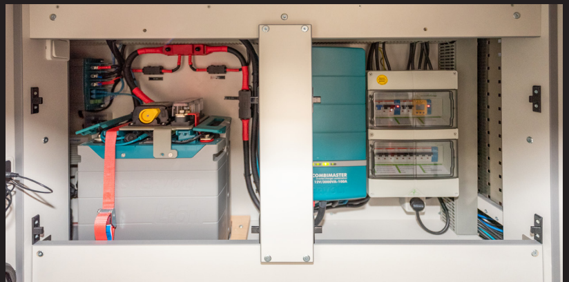
Zuverlässige Energieversorgung mit einer Mastervolt® Lithium-Ionen-Batterie und einem CombiMaster.
